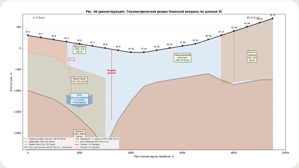
Рис. 46. Геоэлектрический разрез Ононской впадины по данным ЗС
