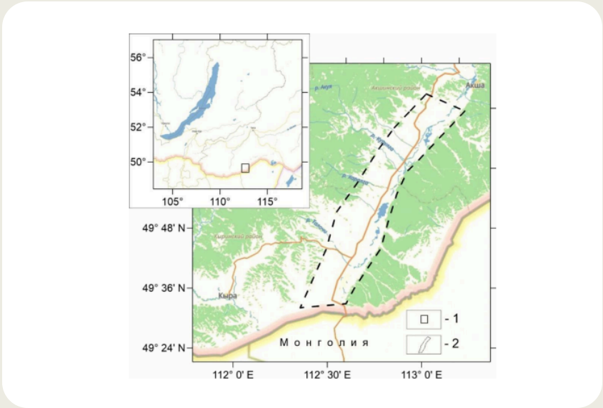
Рис. 1. Схема расположения Ононской впадины: 1 – положение района работ; 2 – границы российской части Ононской впадины.
