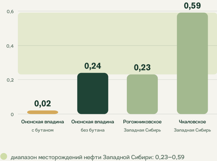
Соотношение ароматических и предельных УВ ( C_{аром}/C_{пред} ): Ононская впадина vs месторождения Западной Сибири
