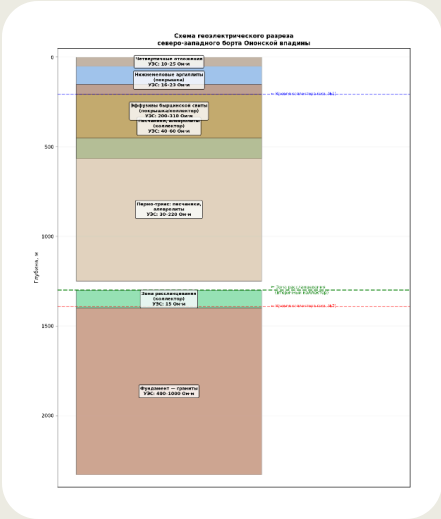
Схема геоэлектрического разреза северо-западного борта Ононской впадины
