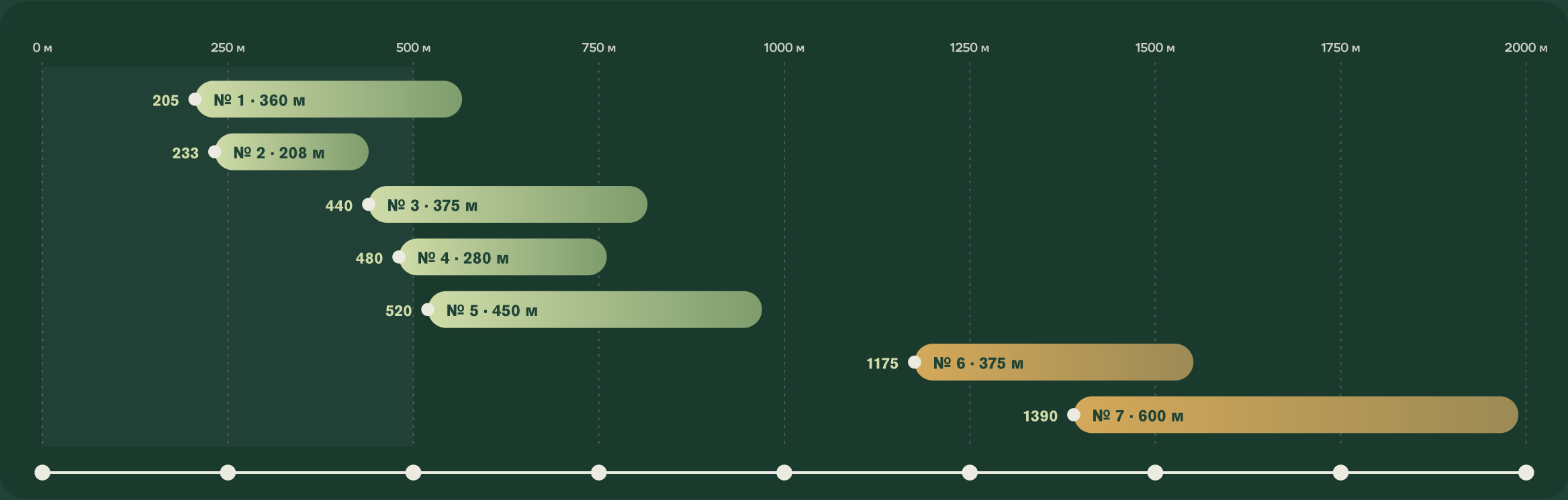
Рис. 6. Перспективные участки заложения поисковых скважин: точка — глубина до кровли коллектора, полоса — мощность коллекторов, м. ● мелкое залегание (до 500 м) ● глубокое залегание
