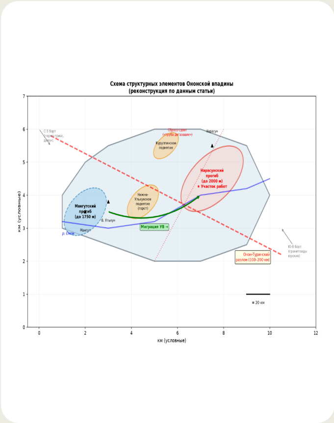
Рис. 1а. Схема структурных элементов Ононской впадины
