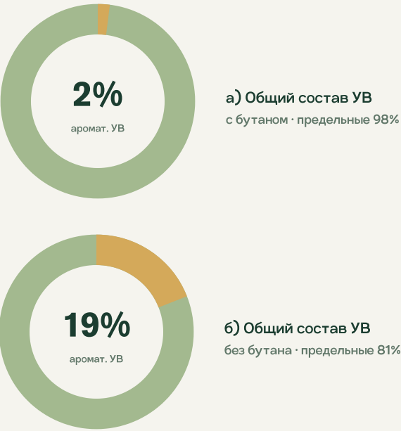
Рис. 3. Суммарный углеводородный состав проб грунта
