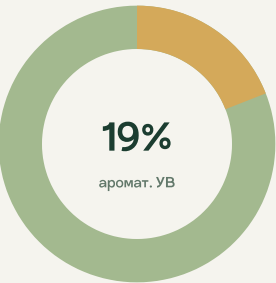
б) Общий состав УВ без бутана • предельные 81%
