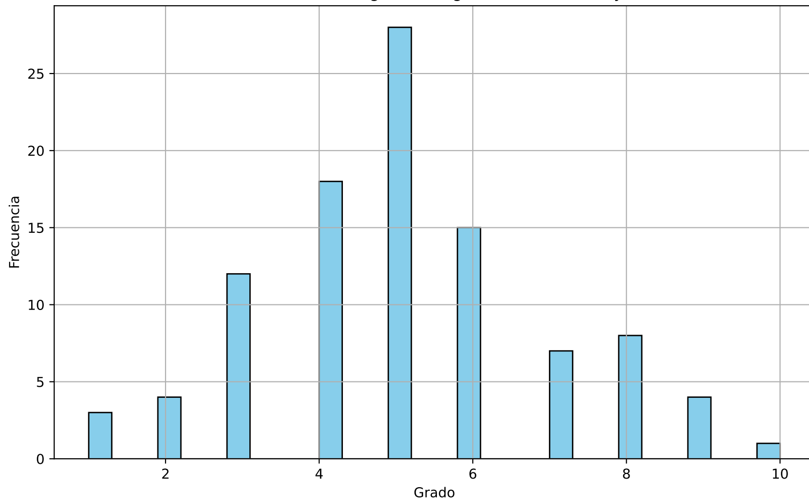
Distribución del grado del grafo - 100 nodos CyL
