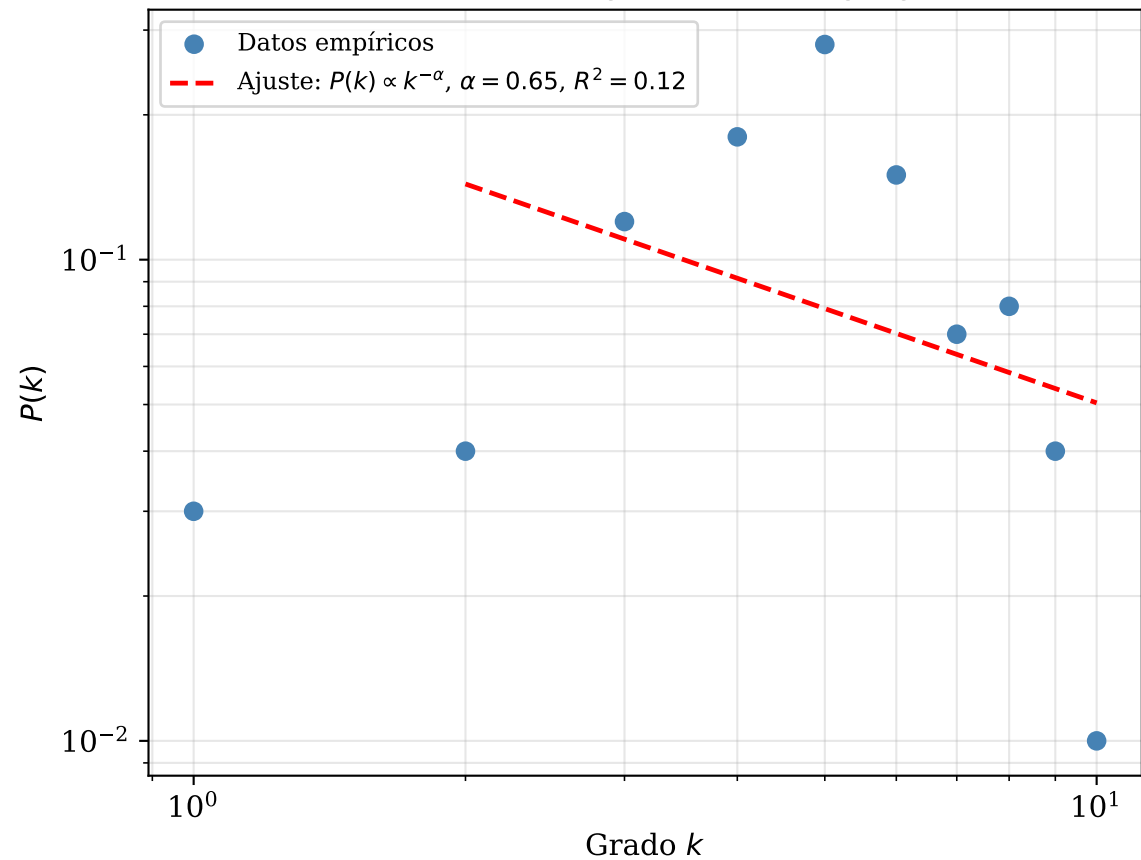
Distribución de grado (escala log-log)
