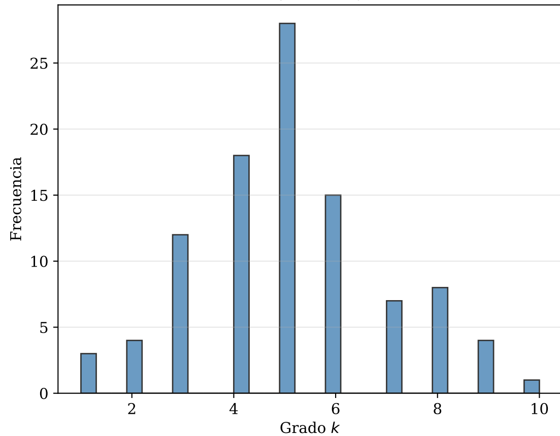
Distribución del grado — CyL (100 nodos)
