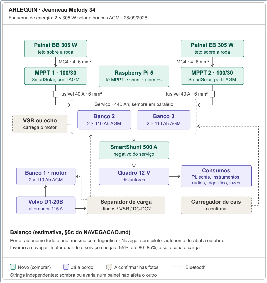
Esquema de energia (28/09/2026): strings independentes, um MPPT por painel, fusível de 40 A à saída de cada um, SmartShunt no negativo do serviço.
