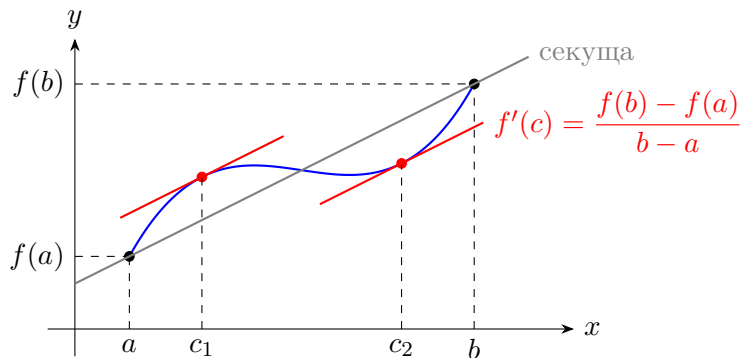
Фигура 2: Геометричен смисъл на теоремата на Лагранж — теоремата гарантира поне една точка c ; в примера са видими две: c_1 и c_2
