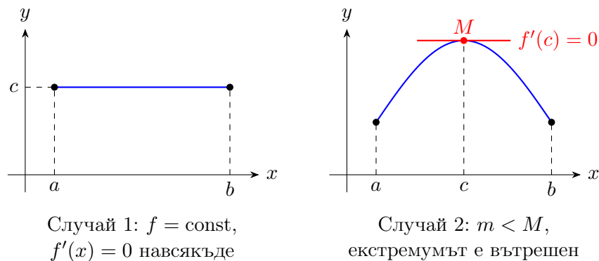
Фигура 1: Геометричен смисъл на теоремата на Рол — Случай 1: f = \text{const} , f' \equiv 0 ; Случай 2: екстремумът се достига във вътрешна точка c , откъдето f'(c) = 0
