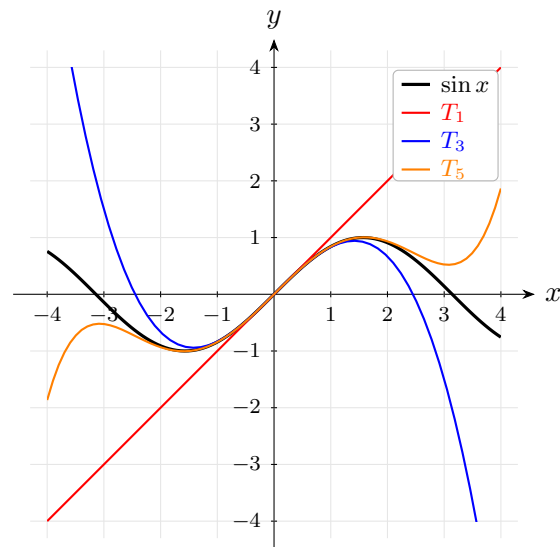
Фигура 4: Приближения на Тейлър за \sin x около x_0 = 0 : T_1 = x ; T_3 = x - \frac{x^3}{6} ; T_5 = x - \frac{x^3}{6} + \frac{x^5}{120}
