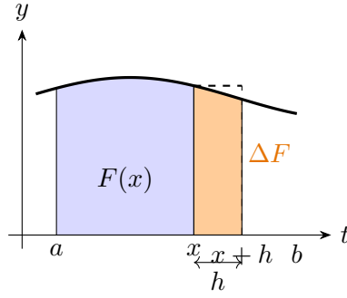
Фигура 3: Геометричен смисъл на F(x) = \int_a^x f(t)dt
