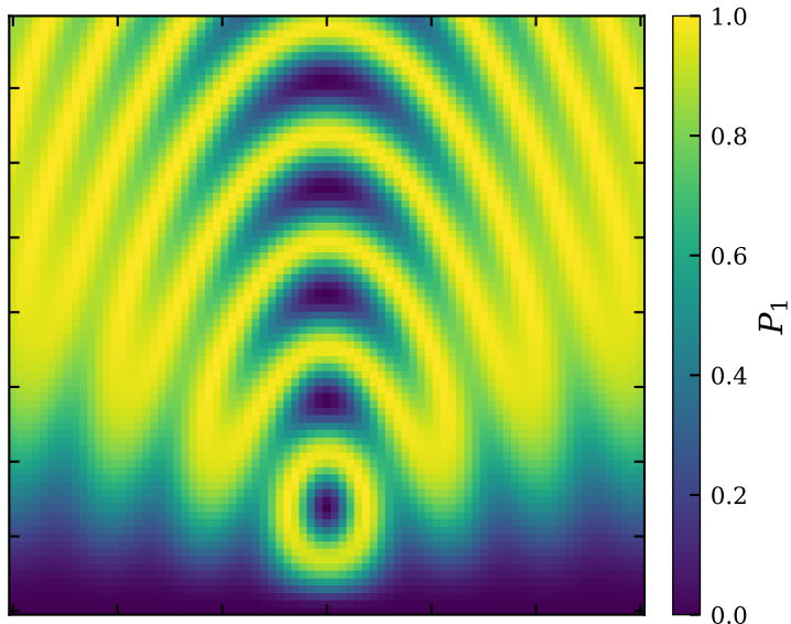
(f) cosine LMSZ + DRAG leakage
