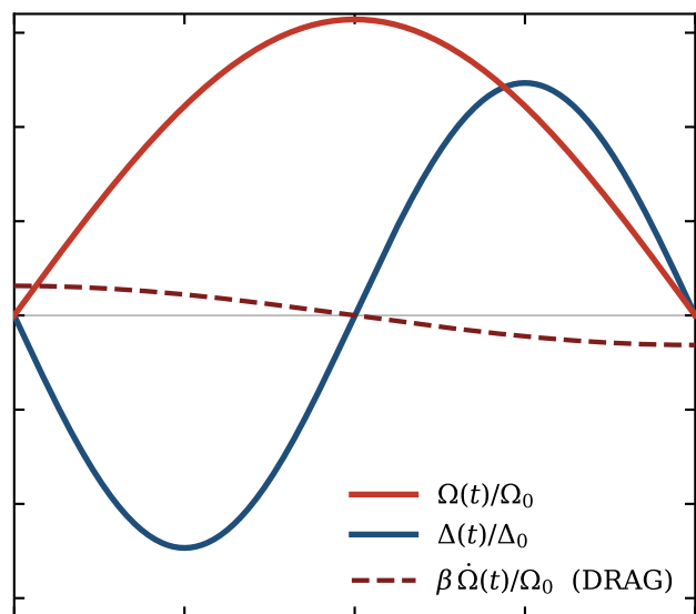
(d) cosine LMSZ + DRAG P_1
