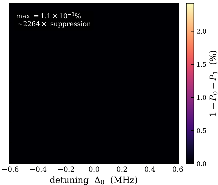
(f) cosine LMSZ + DRAG leakage
