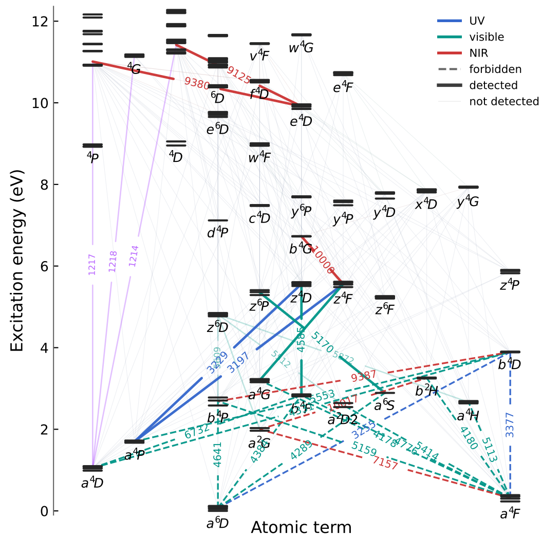
Optical: 4-6 eV \rightarrow 2-4 eV
