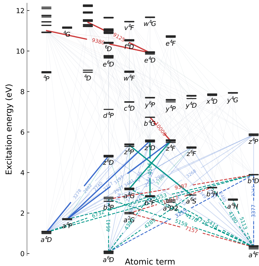
UV: 4-6 eV \rightarrow 0-2 eV
