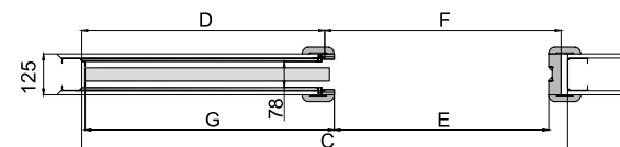
TABULKA ROZMĚROVÁ [mm] / TABUĽKA ROZMEROVÁ [mm]
