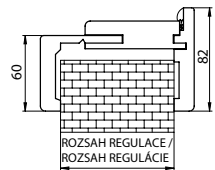
Tloušťka ostění nadpraží - 16 mm / Hrúbka ostenia nadpražie - 16 mm
