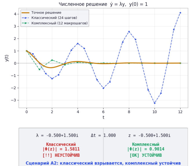
Рисунок 12 – Сценарий A2: \lambda = -0,5 + 1,5i , \Delta t = 1,0 . Классический Эйлер показывает растущие осцилляции ( |\Phi| = 1,58 ), комплексный 2-шаговый плавно затухает ( |\Phi| = 0,90 ). Это и есть «практическое расширение» области устойчивости за счёт перехода в комплексную плоскость.
