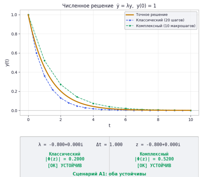
Рисунок 11 – Сценарий A1: \lambda = -0,8 , \Delta t = 1,0 . Оба метода устойчивы ( |\Phi_{classic}| = 0,20 ; |\Phi_{complex}| = 0,52 ). Численные кривые отлично согласуются с точным e^{\lambda t} .
