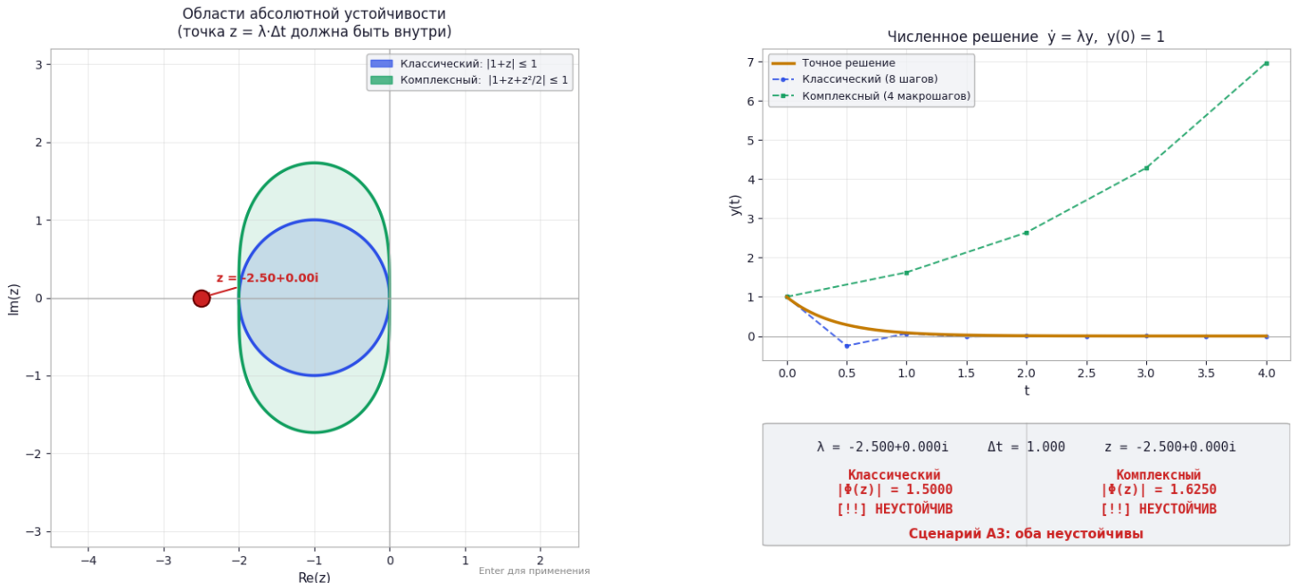
Рисунок 13 – Сценарий А3: \lambda = -2,5 , \Delta t = 1,0 . Оба метода неустойчивы. Это напоминает, что для достаточно жёстких задач даже комплексный путь не спасает – нужен другой способ (например, неявный или с уменьшением \Delta t ).
