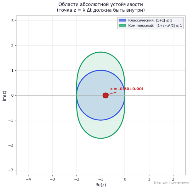
Рисунок 11 – Сценарий A1: \lambda = -0,8 , \Delta t = 1,0 . Оба метода устойчивы ( |\Phi_{classic}| = 0,20 ; |\Phi_{complex}| = 0,52 ). Численные кривые отлично согласуются с точным e^{\lambda t} .
