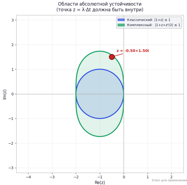
Рисунок 12 – Сценарий A2: \lambda = -0,5 + 1,5i , \Delta t = 1,0 . Классический Эйлер показывает растущие осцилляции ( |\Phi| = 1,58 ), комплексный 2-шаговый плавно затухает ( |\Phi| = 0,90 ). Это и есть «практическое расширение» области устойчивости за счёт перехода в комплексную плоскость.
