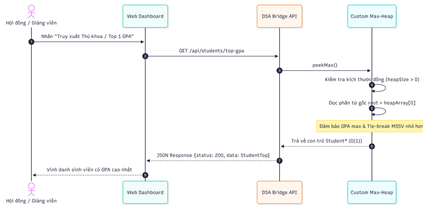
Hình 9. Sơ đồ tuần tự (Sequence Diagram) luồng trích xuất GPA cao nhất trên Max-Heap
