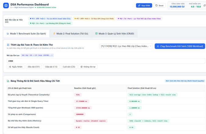
Hình 23. Benchmark RQ1 khi tra cứu mã lớp không tồn tại
