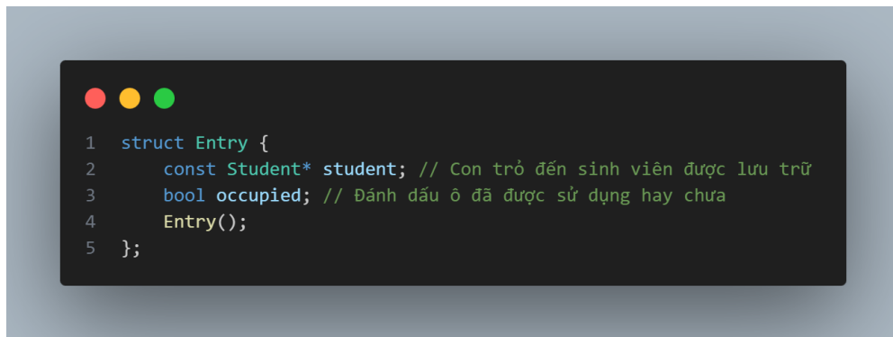
Hình 2. Cấu trúc ô nhớ Entry trong Bảng băm
