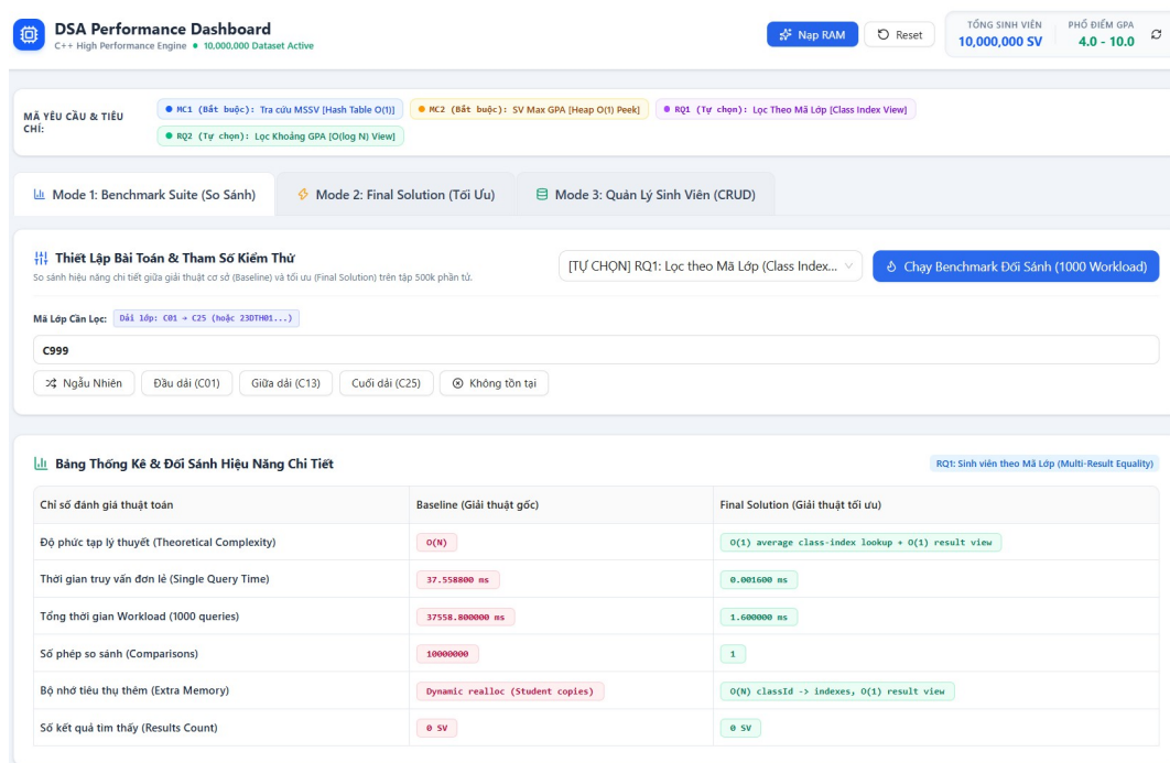
Figure 23. Benchmark RQ1 khi tra cứu mã lớp không tồn tại
