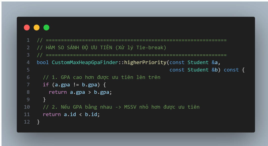
Figure 10. Hiện thực toán tử phân định đồng hạng kết hợp GPA và MSSV
