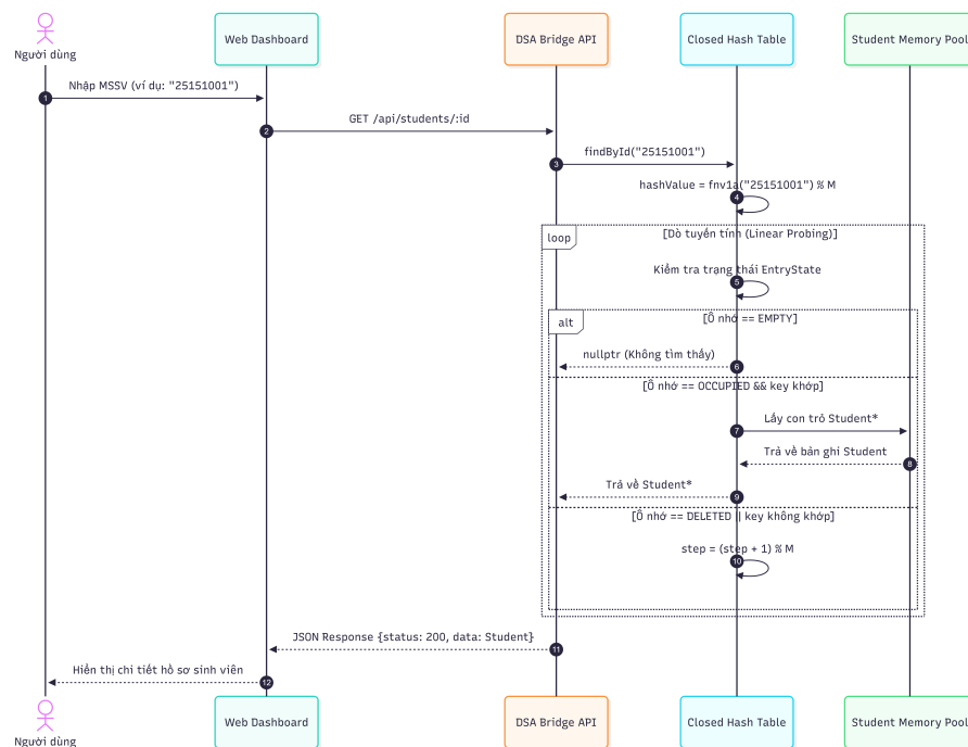
Figure 6. Sơ đồ tuần tự (Sequence Diagram) luồng tra cứu chính xác theo MSSV trên Bảng băm
