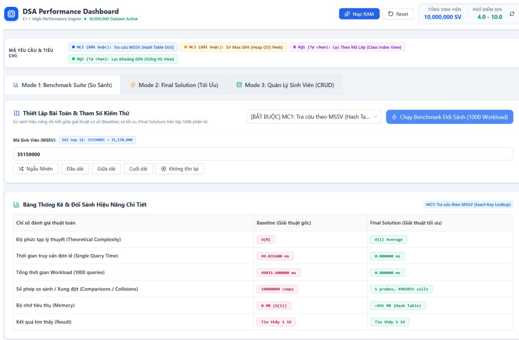
Figure 17. Benchmark MC1 tra cứu MSSV tại cuối dải dữ liệu
