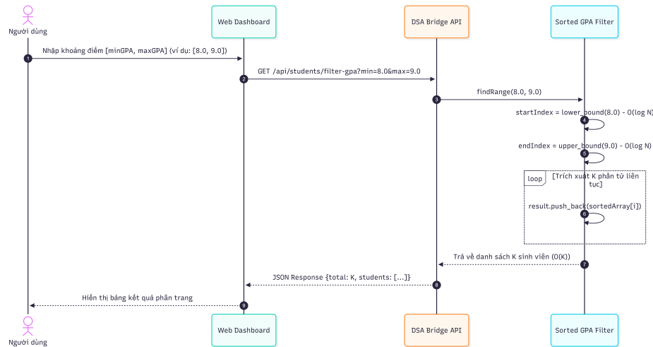
Figure 13. Sơ đồ tuần tự (Sequence Diagram) luồng lọc sinh viên theo khoảng GPA
