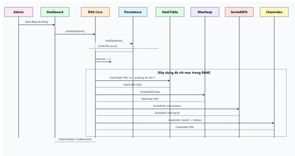
Figure 14. Sơ đồ tuần tự (Sequence Diagram) luồng khởi tạo và nạp dữ liệu hàng loạt (Bulk Load)
