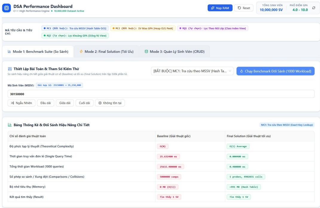
Figure 16. Benchmark MC1 tra cứu MSSV tại giữa dải dữ liệu
