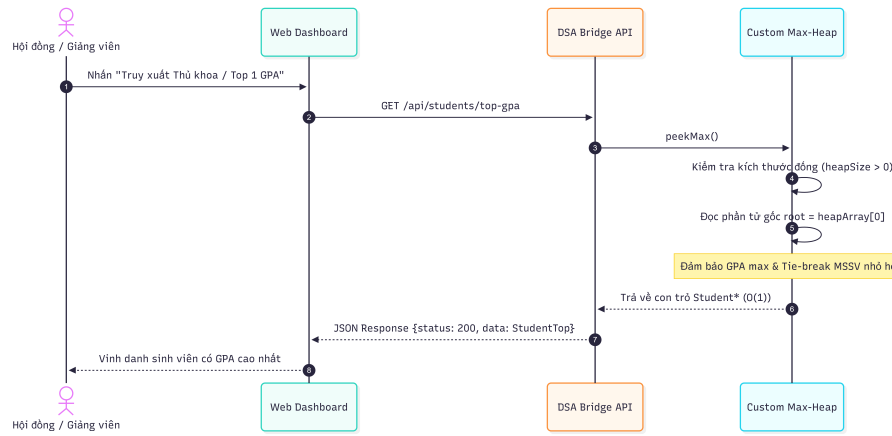
Figure 9. Sơ đồ tuần tự (Sequence Diagram) luồng trích xuất GPA cao nhất trên Max-Heap
