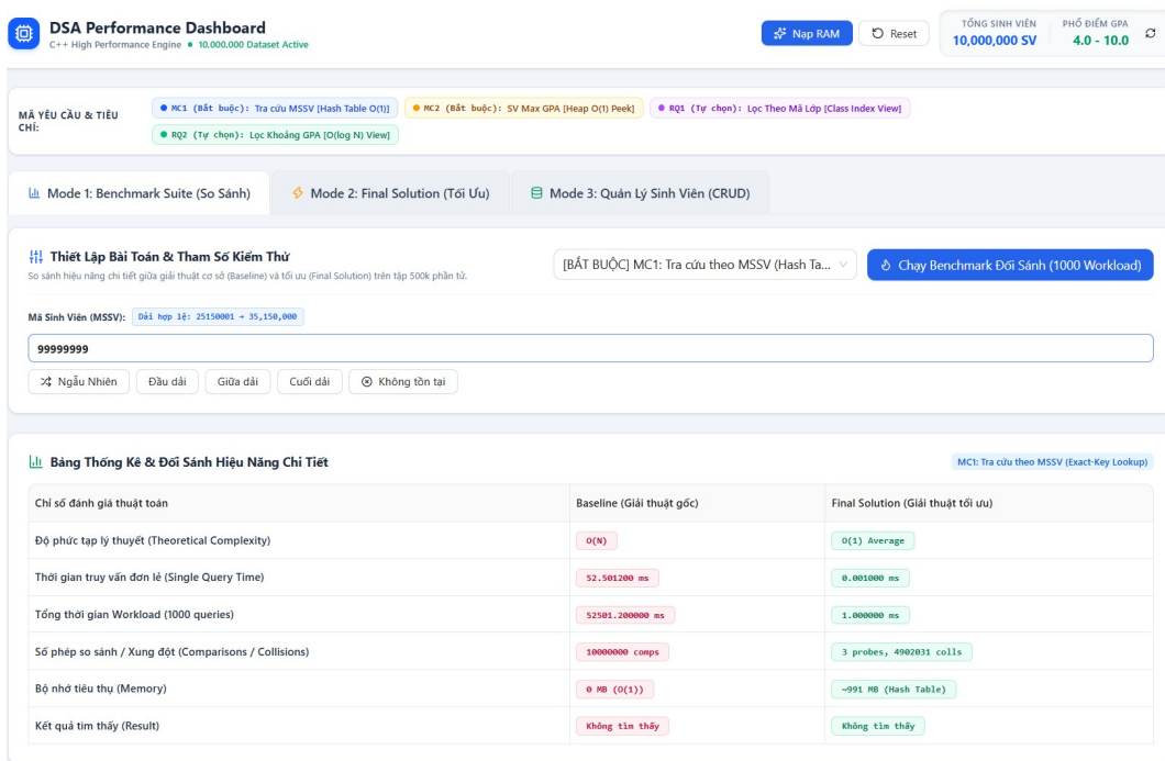
Figure 18. Benchmark MC1 tra cứu MSSV khi khóa không tồn tại trong hệ thống
