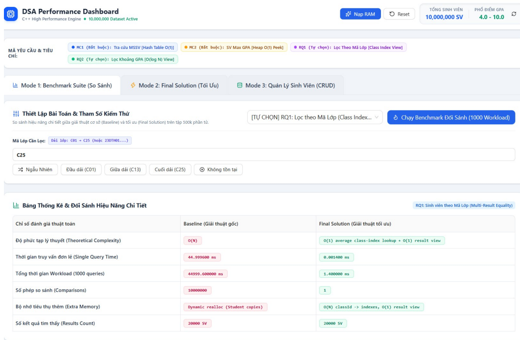
Figure 22. Benchmark RQ1 lọc danh sách sinh viên lớp C25 (Cuối dài)
