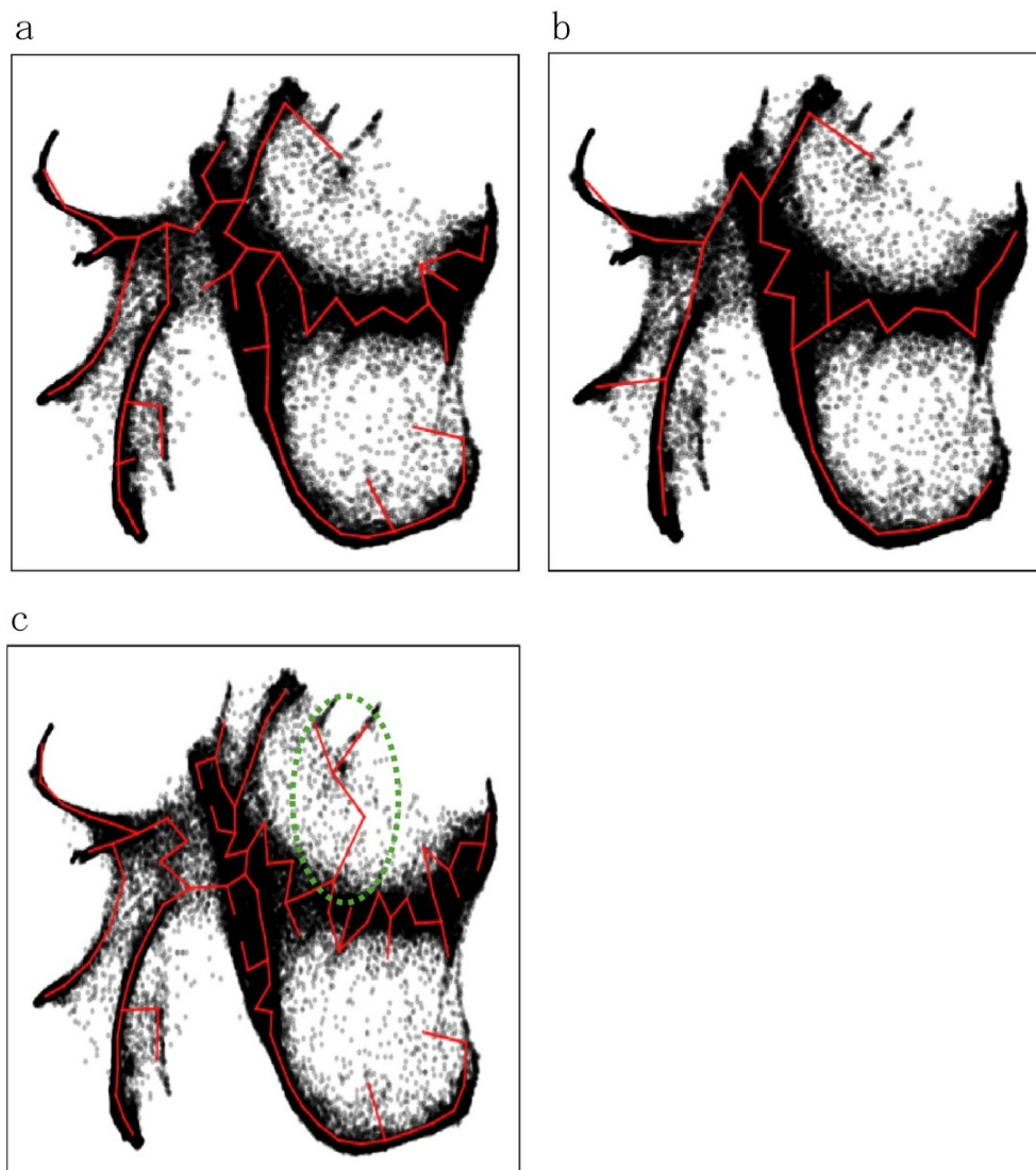
図 14: クラスタ数による最小全域木の比較図。Hematopoiesis のデータを使用している。a クラスタ数 76 b クラスタ数 35 c クラスタ数 100
