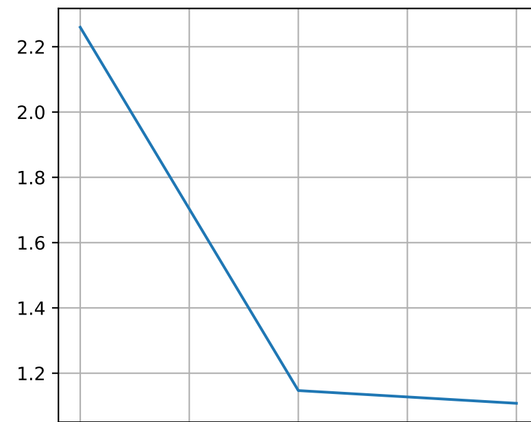
TrainMask
