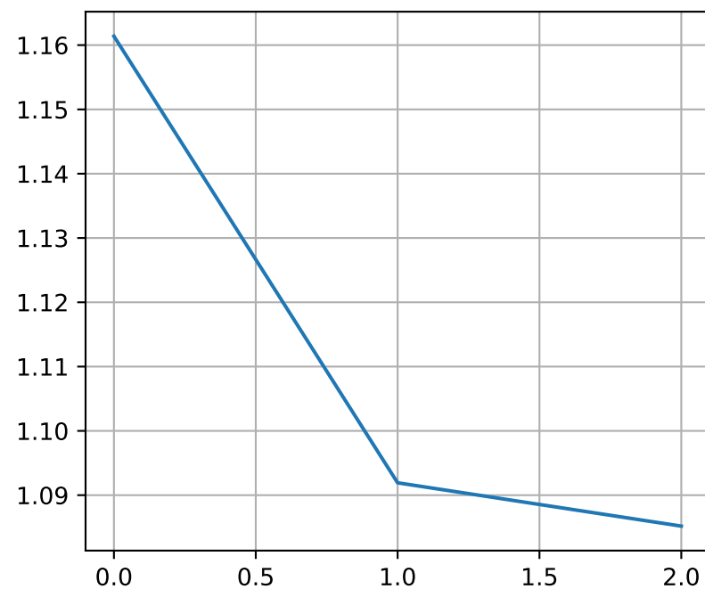
ValTotal
