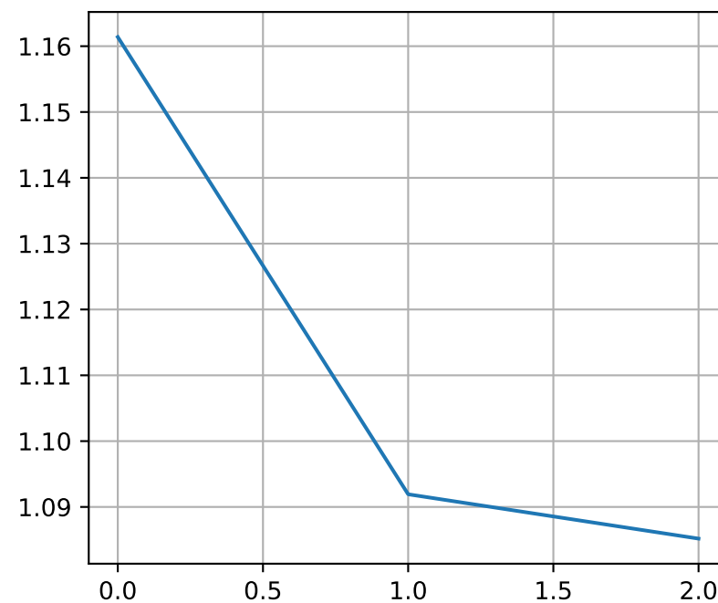
ValMask
