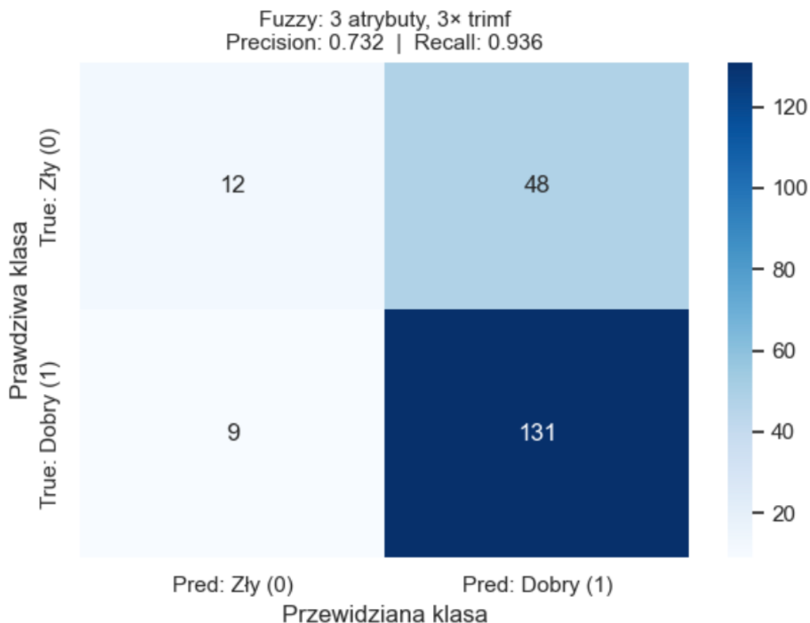
Rysunek 4. Macierz pomyłek dla najlepszej konfiguracji systemu rozmytego (3 atrybuty, 3× trimf)
