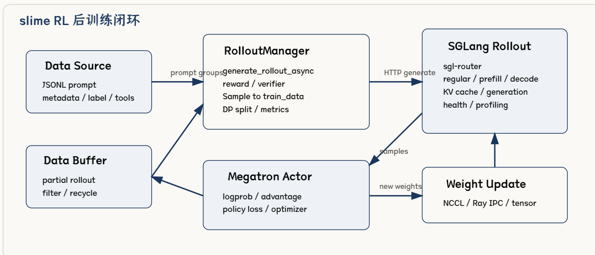
图 1: slime 的主控制闭环。图中箭头表示数据或权重的主要流向, 真实实现中由 Ray actor、HTTP server、NCCL group 和本地进程共同完成。
