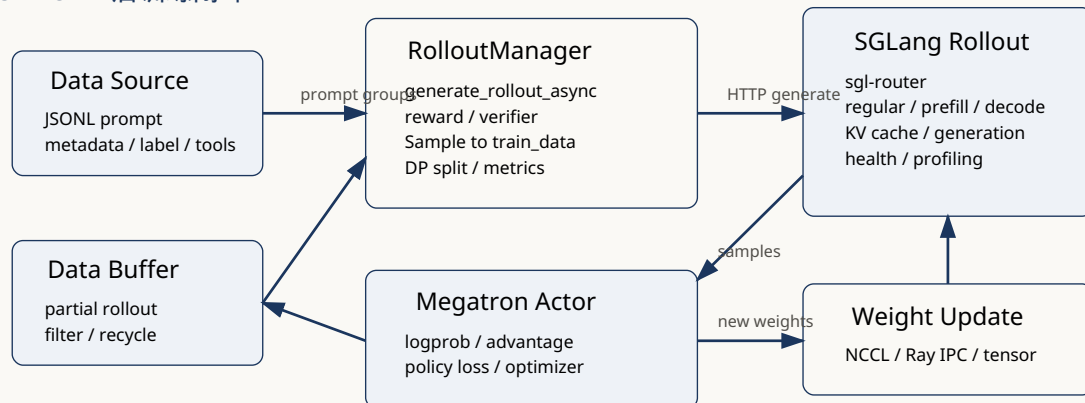
slime RL 后训练闭环
