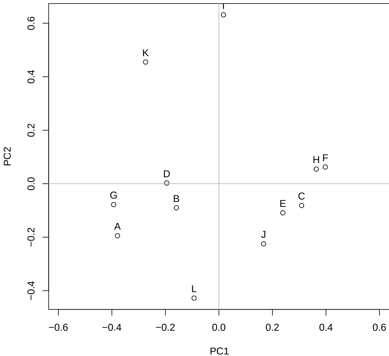
PC scores: PC1-PC2
