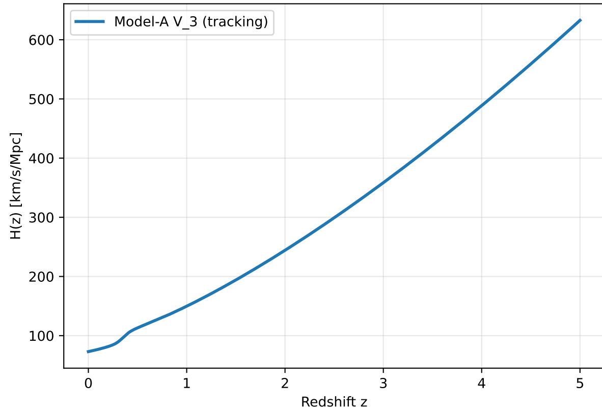
Hubble parameter (Model-A, H_0 = 73.04 )
