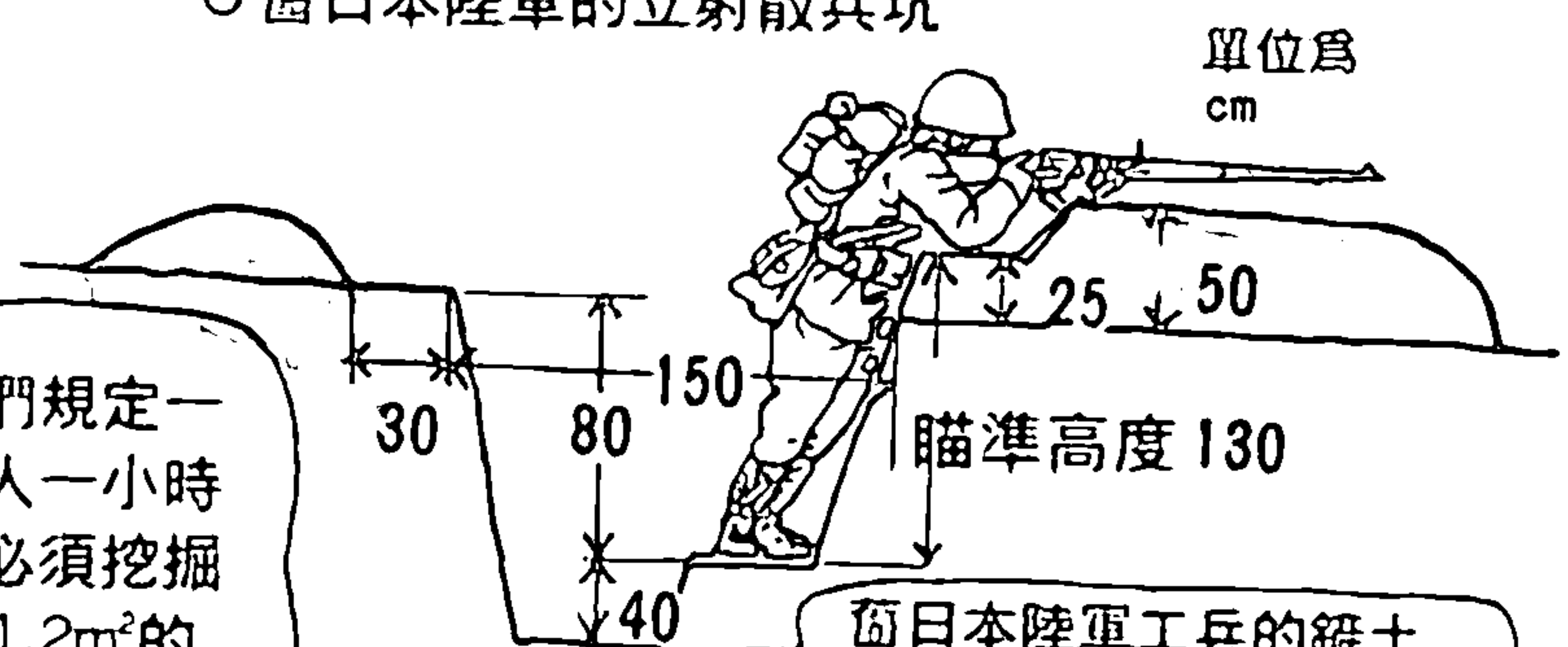
○舊日本陸軍的立射散兵坑
