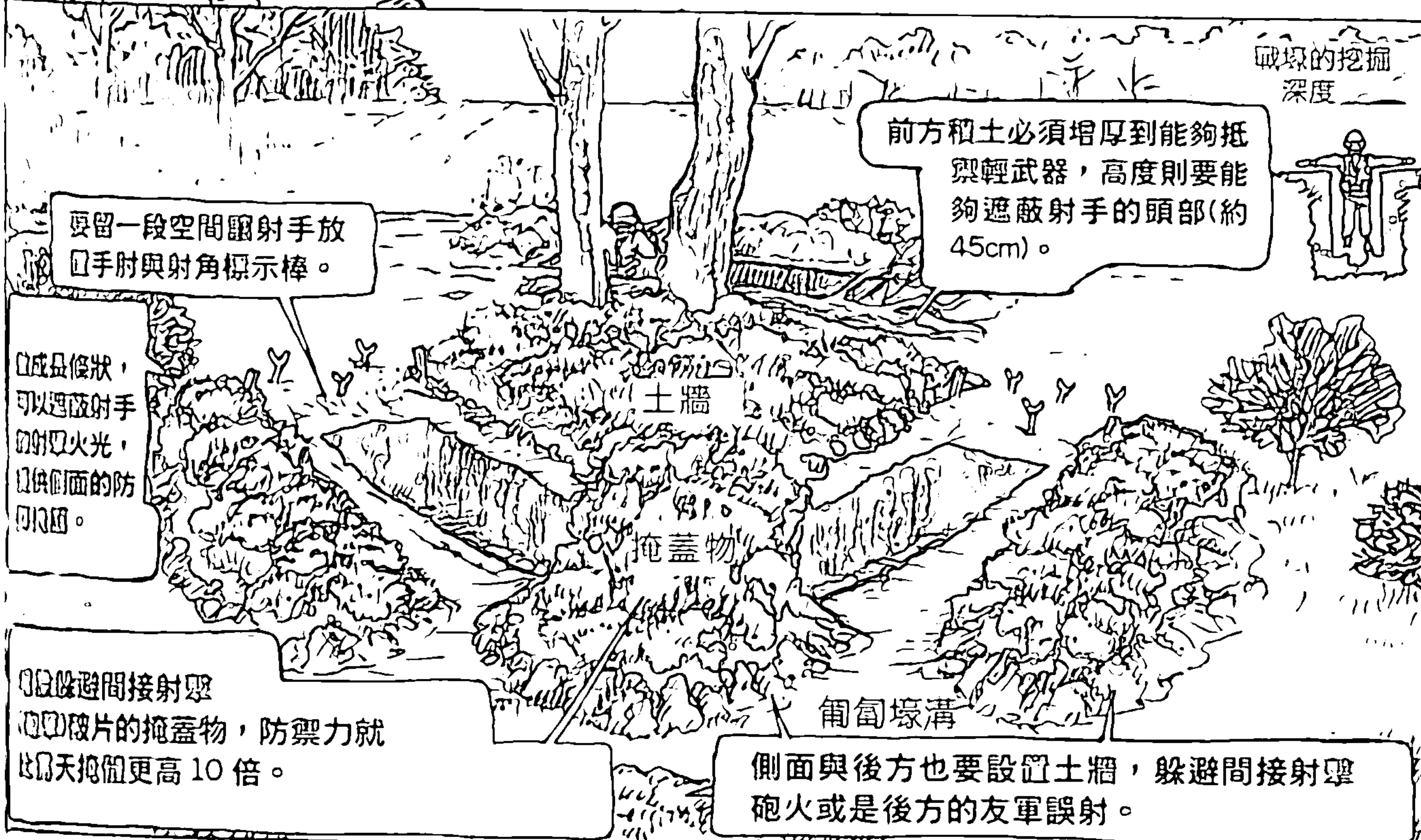
雙人戰鬥掩體
