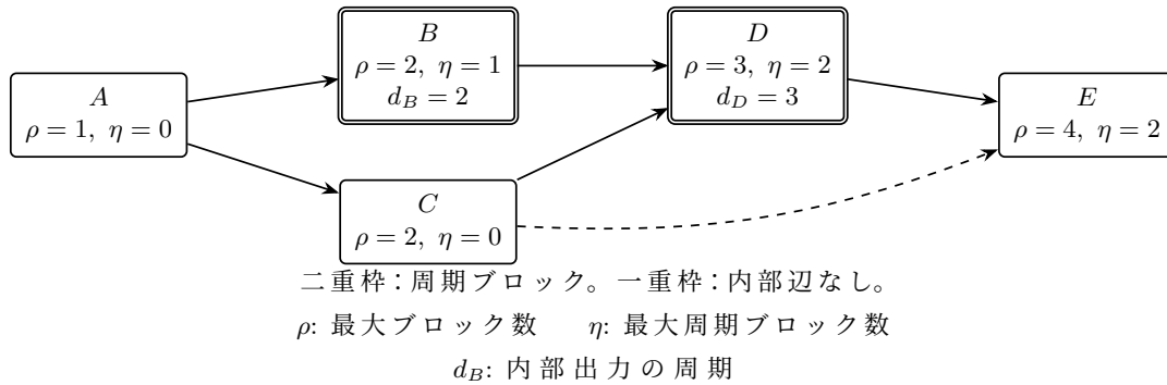
SCC 凝縮 DAG の概念例 (実計算グラフ全体ではない)
