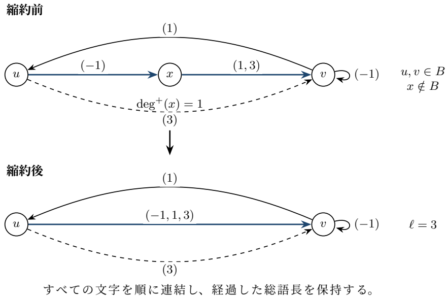
図 5. 正確な縮約の例。頂点 x の出辺は一本であり、 u と v はそれぞれ二本の出辺を持つためマクロ頂点である。語 (-1) と (1, 3) は (-1, 1, 3) に連結され、その語長は三のまま保たれる。他の辺はすべて保持される。線種で対応する辺を示す。
