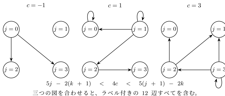
図 7. K = 4 における 5/2 初期グラフの全十二辺を、キャリー c ごとの三図に分けて示す。各図の四頂点は共通であり、三図を重ねるとグラフ全体になる。辺は図の下に記した厳密な整数不等式から列挙され、表 5 と一致する。
