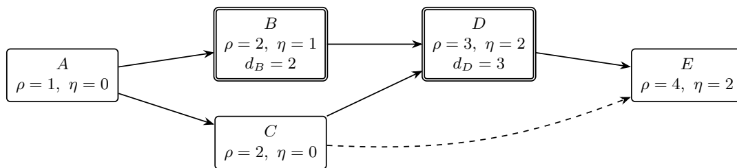
SCC 凝縮 DAG の概念例 (実計算グラフ全体ではない)
