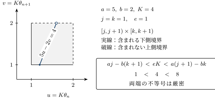
図 2. a = 5, b = 2, K = 4, j = k = 1, e = 1 におけるセル整合条件。直線は半開正方形と、 u = (4 + 2v)/5, 1 \leq v < 2 の部分で交わる。下端は含まれ、上端は含まれない。セル対の判定は局所的であり、軌道全体の存在を主張するものではない。
