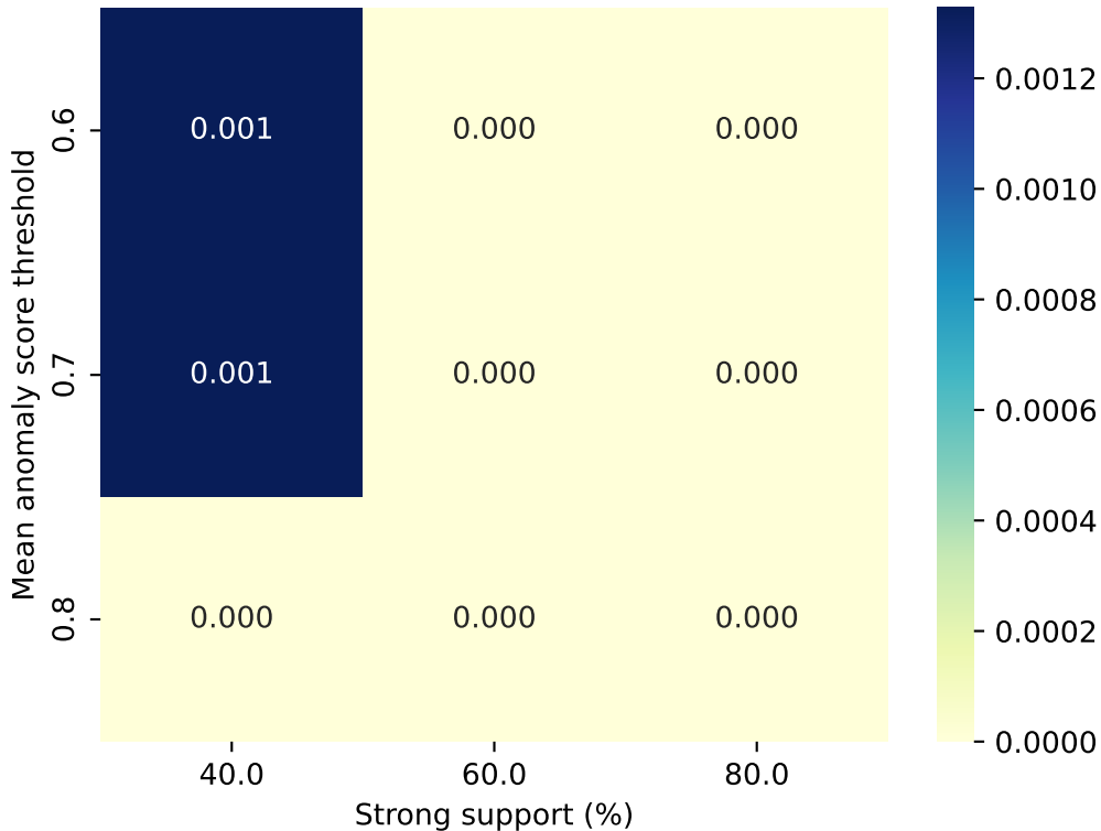
Selective Weak Promotion — F1 (DBSCAN sub-clusters)
