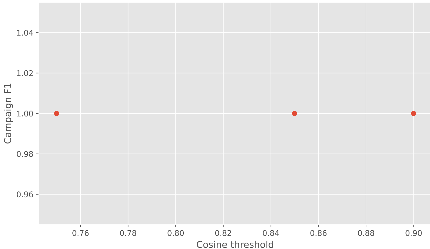
strong_campaign: campaign F1 vs edge threshold
