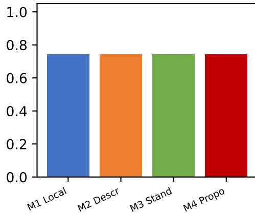
f1
