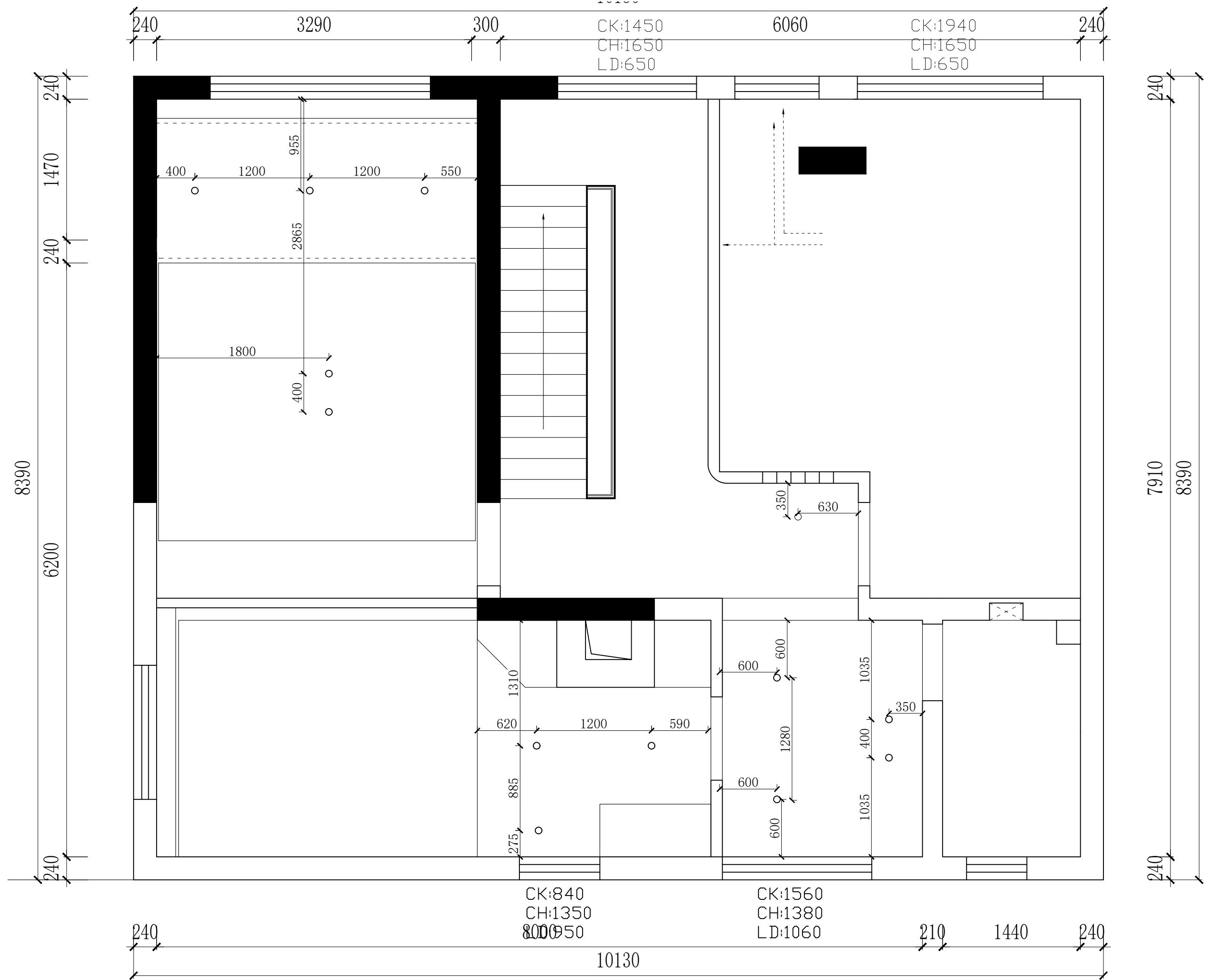
⊗ 二层顶棚布置图
