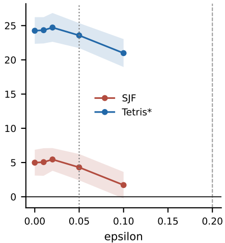
P3 FGSM
