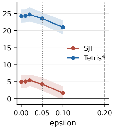
P3 FGSM
