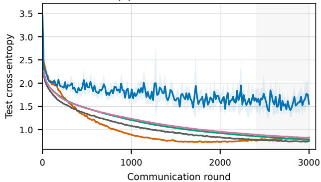
(d) CIFAR-10 ResNet-14
