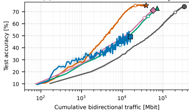
(d) ResNet-14 communication efficiency
