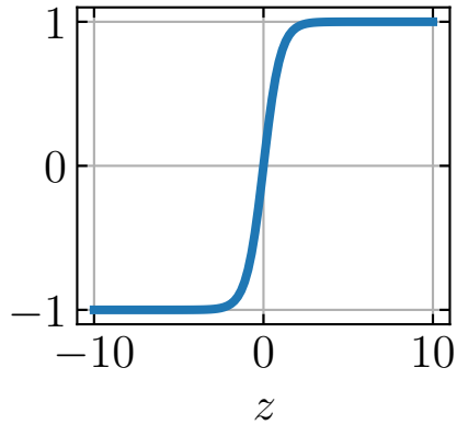
Tanh
