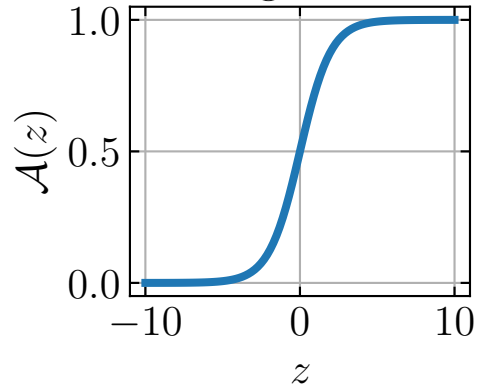
Sigmoid
