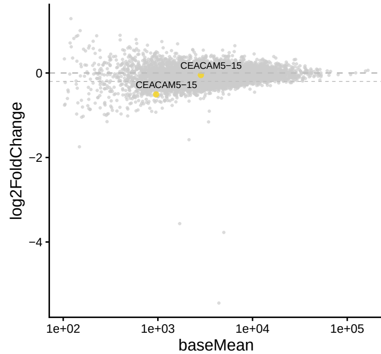
CEACAM5-15 | Cluster vs UT
