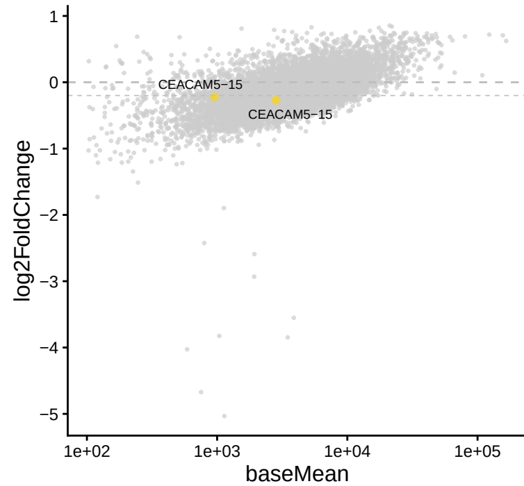
CEACAM5-15 | UT vs B
