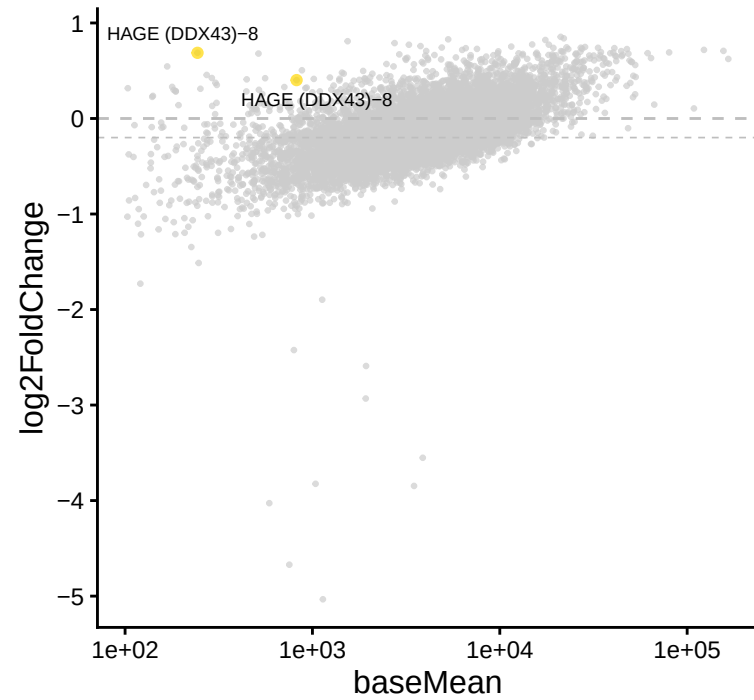
HAGE (DDX43)-8 | UT vs B
