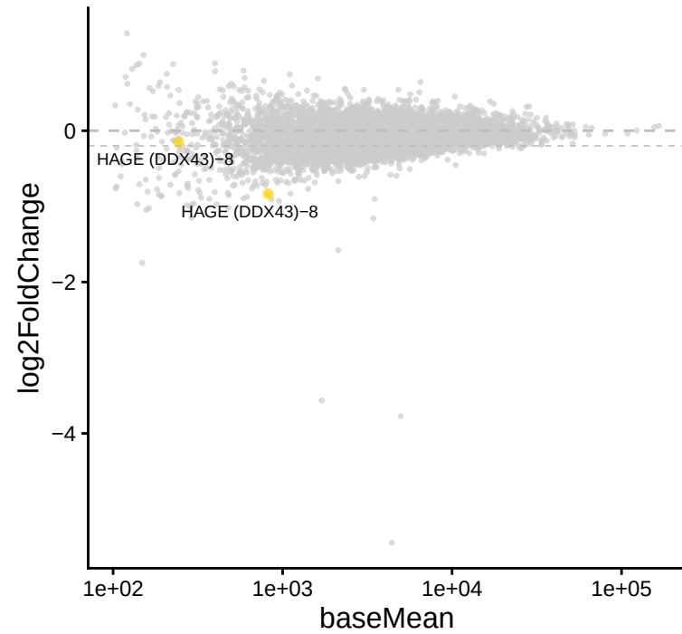
HAGE (DDX43)-8 | Cluster vs UT
