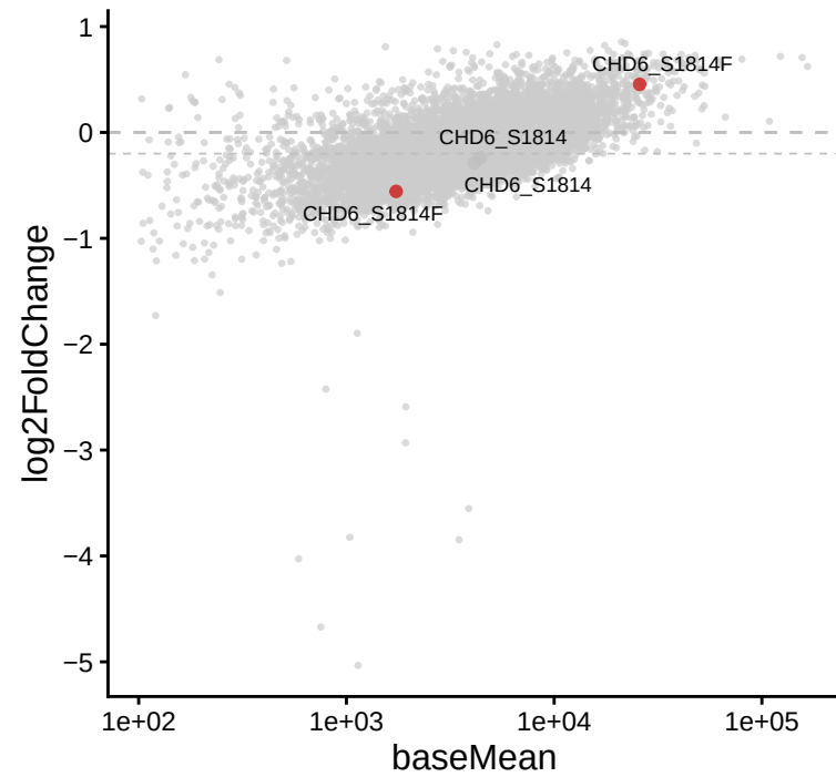
CHD6_S1814F | UT vs B
