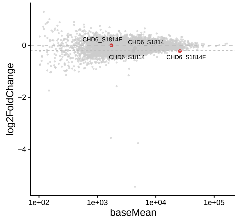
CHD6_S1814F | Cluster vs UT
