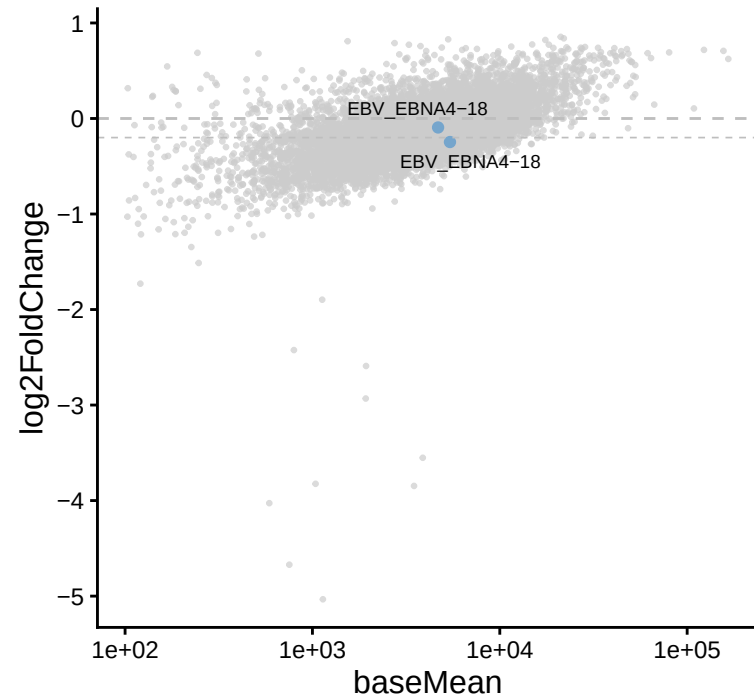
EBV_EBNA4-18 | UT vs B
