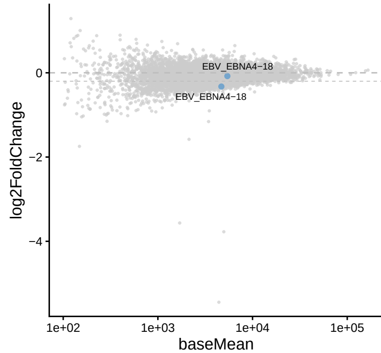
EBV_EBNA4-18 | Cluster vs UT
