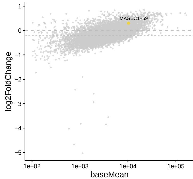
MAGEC1-59 | UT vs B
