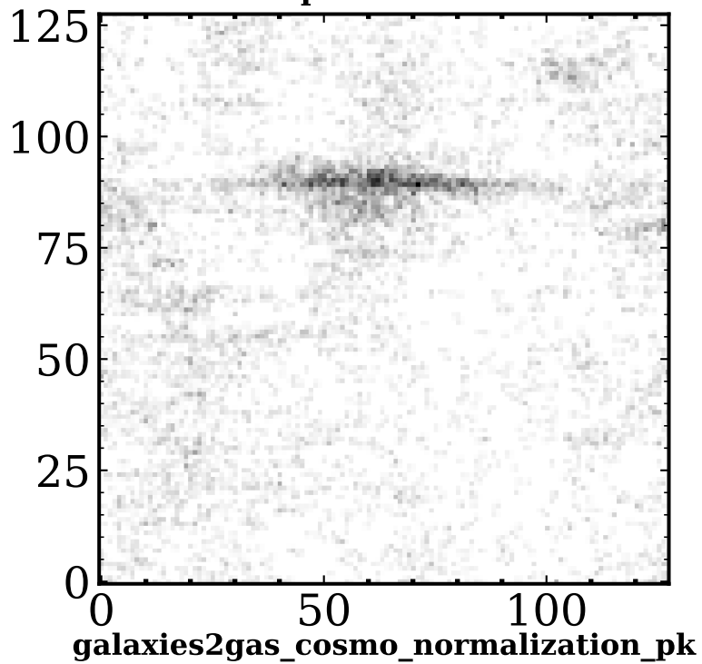
Input Galaxies
