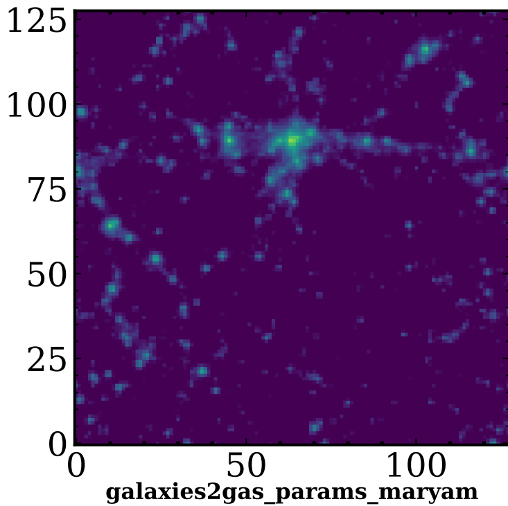
True DM
