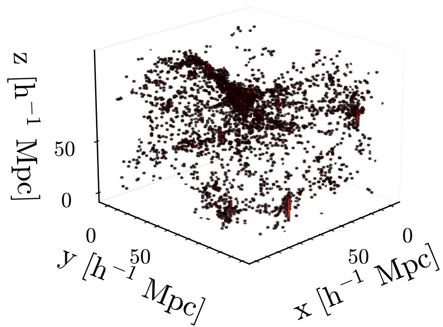
Input Galaxies
