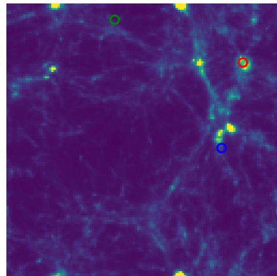
Posterior Sample
