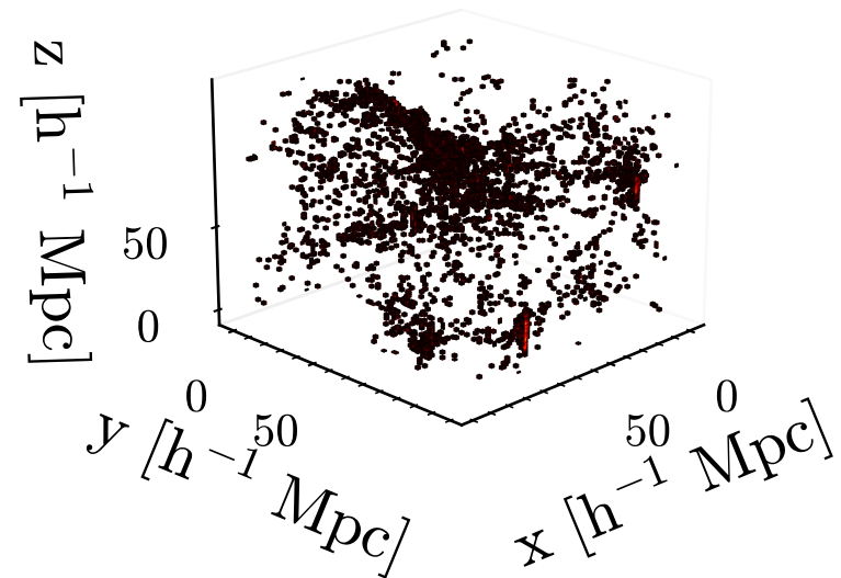
Input Galaxies
