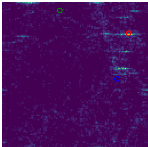
Input galaxies
