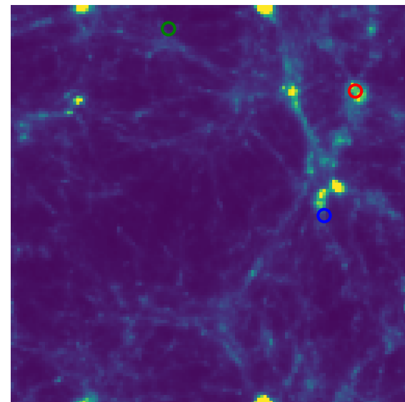
Posterior Sample
