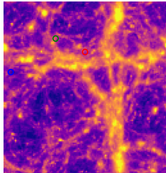
Posterior Sample
