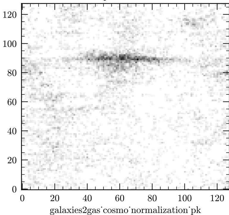
Input Galaxies
