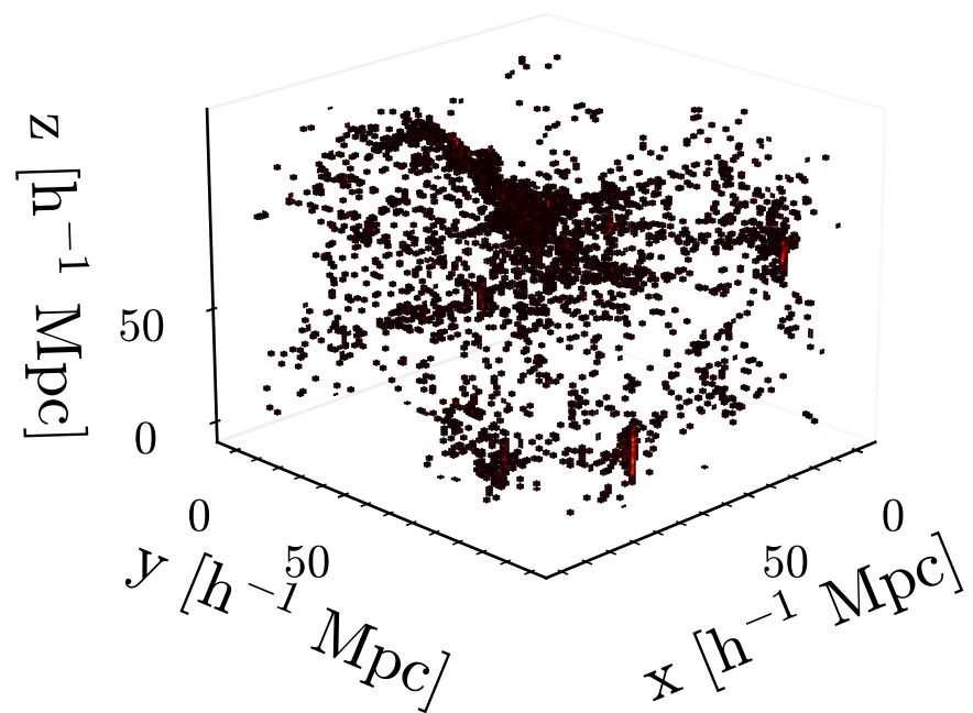
Input Galaxies
