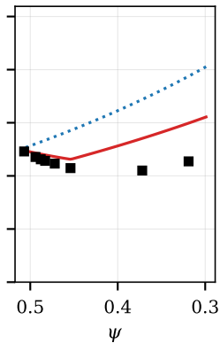
(d) NMC811
